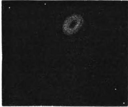
FIG. 42. 57 M. LYRÆ.
