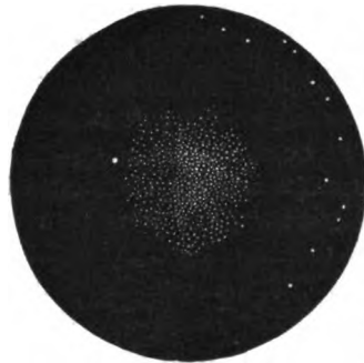
FIG. 43. 56 M. LYRÆ.
