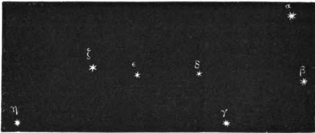
FIG. 17. URSA MAJOR.
