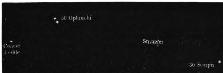
FIG. 35. 36 OPHIUCHI.
