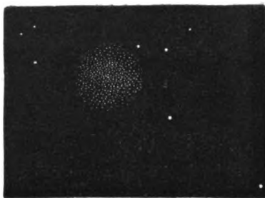
FIG. 47. 2 M. AQUARIJ.
